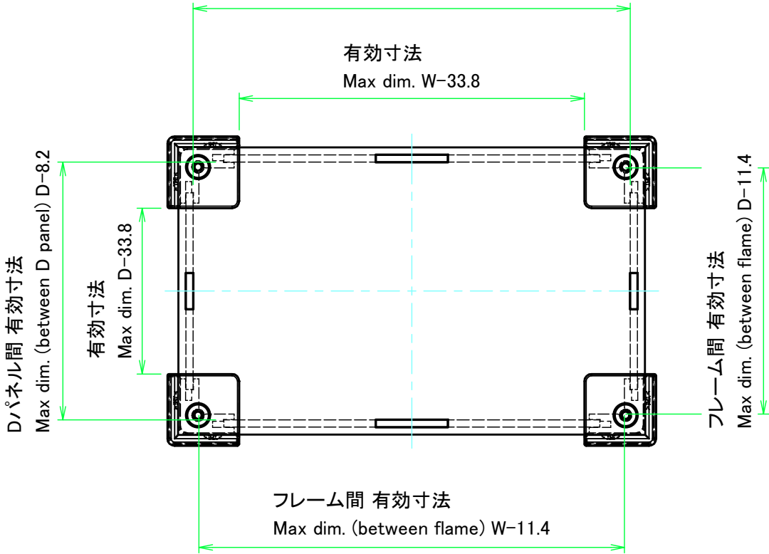
Wパネル間 有効寸法 Max dim. (between W panel) W-8.2
